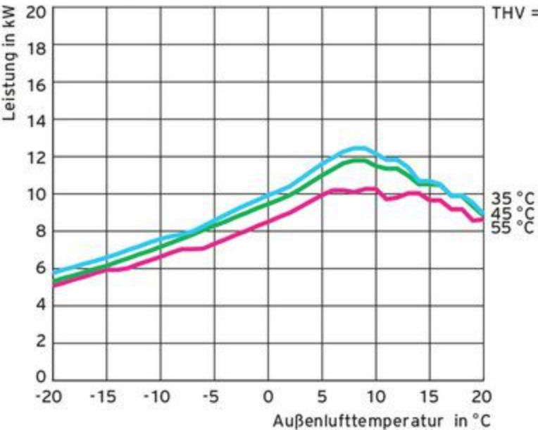
Leistungsdiagramm VWL 75/6 A S2
